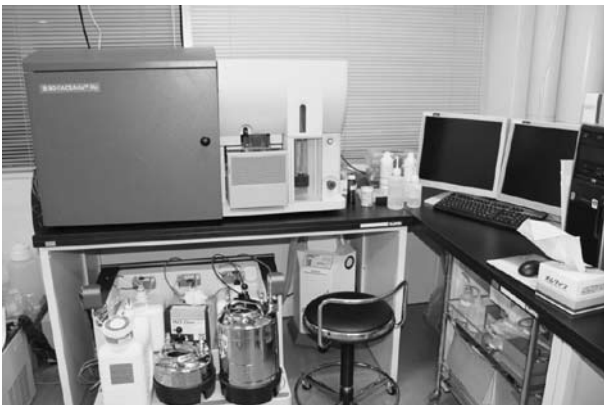
図8 . セルソーター ( Becton Dickinson FACS Aria II ). 細胞集団の情報を解析すると共に , その情報を基に特定の細胞を生きたまま回収することができる .
