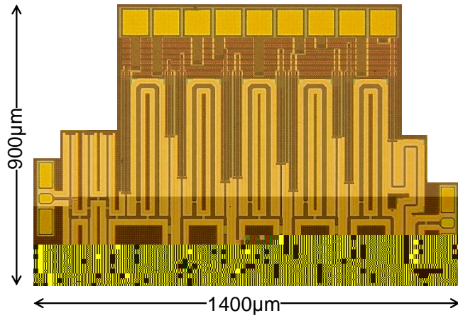
55-nm DDC CMOSプロセスを用いた 0.5V動作W帯増 回 のチップ 真
