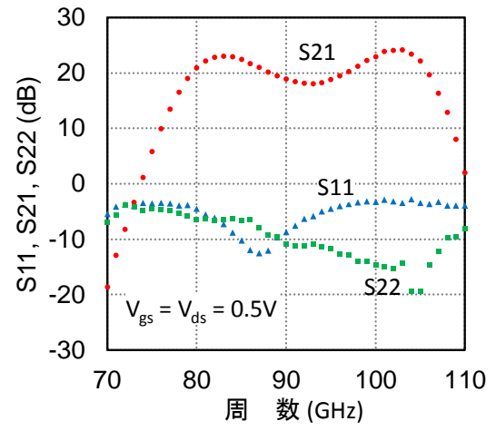
0.5V動作W帯増 回 の 測 果
