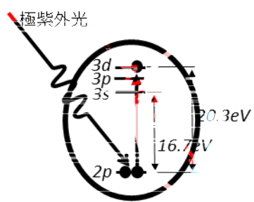
(i) 励起ネオン原子
