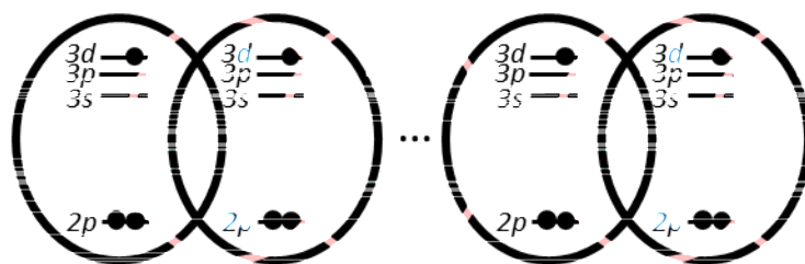
(ii) 多重励起したネオン・クラスター
