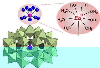
ポリオキソメタレート
