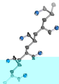
ポリアリルアミン
